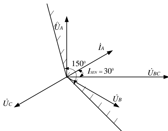
图 3-1-3-1 过流保护方向元件动作特性（阴影部分表示动作区）
