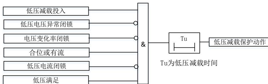
图 3-1-12 低压减载原理框图
