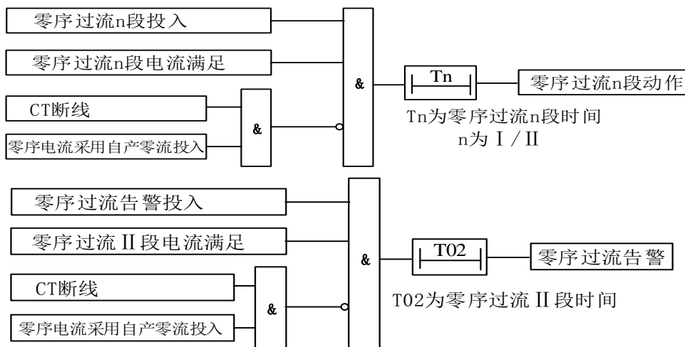
图 3-1-4 零序过流保护原理框图
