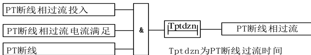
图 3-1-7 PT 断线过流保护原理框图
