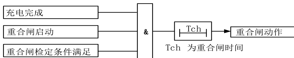
图 3-1-9 重合闸逻辑图
