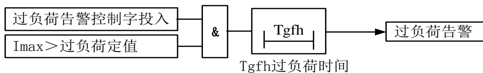
图 3-1-8 过负荷告警原理框图
