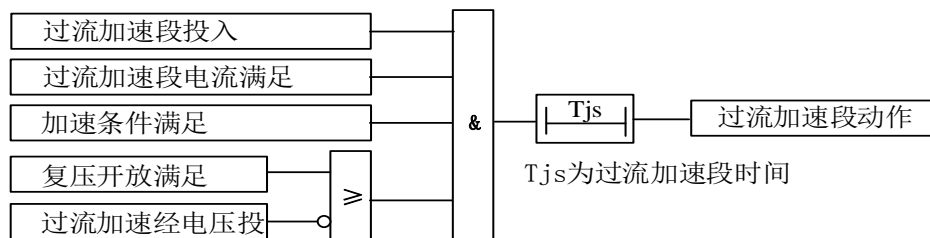
图 3-1-5 过流加速保护原理框图
