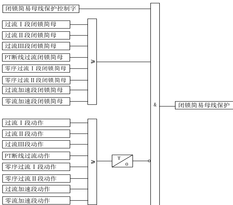
图 3-1-13 闭锁简易母线保护原理框图
