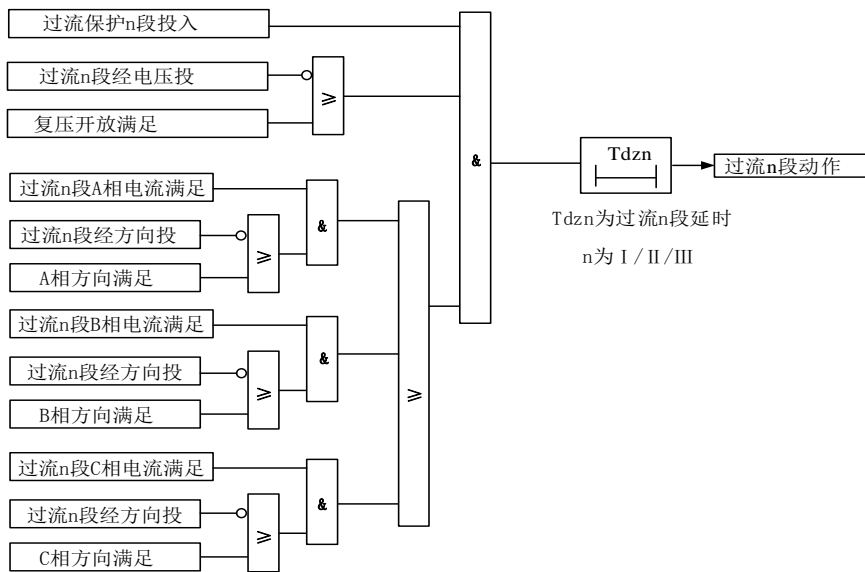
图 3-1-3-2 过流保护原理框图
