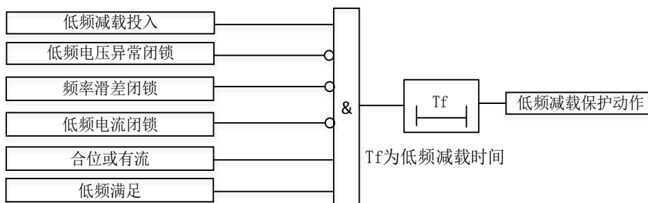
图 3-1-11 低频减载原理框图
