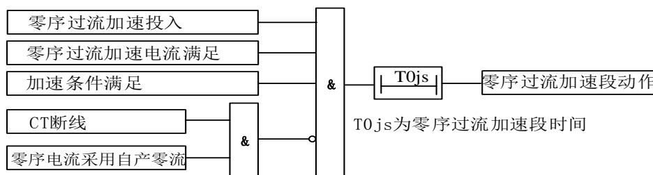
图 3-1-6 零序过流加速保护原理框图
