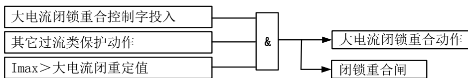
图 3-1-10 大电流闭锁重合闸保护原理框图
