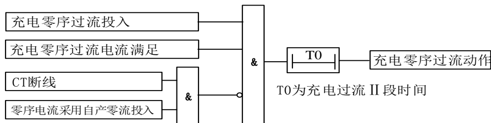
图 3-1-2 充电零序过流保护原理框图
