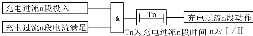
图 3-1-1 充电过流保护原理框图
