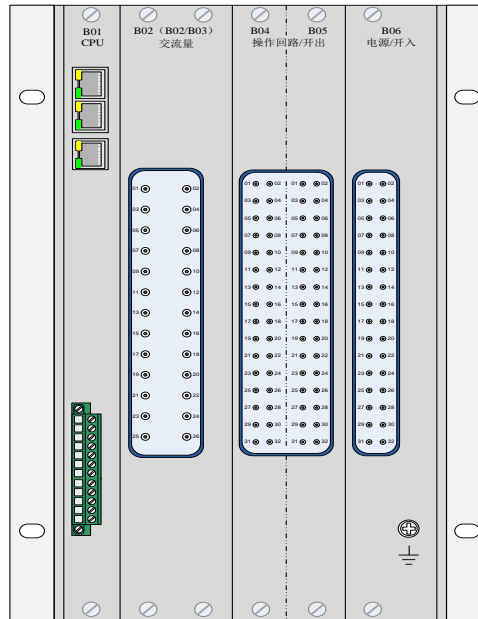
图 4-2-1 装置插件示意图
