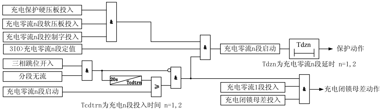
图 3-2 零序过流充电保护原理框图
