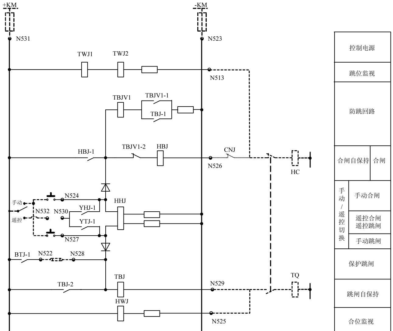
装置操作回路原理图
