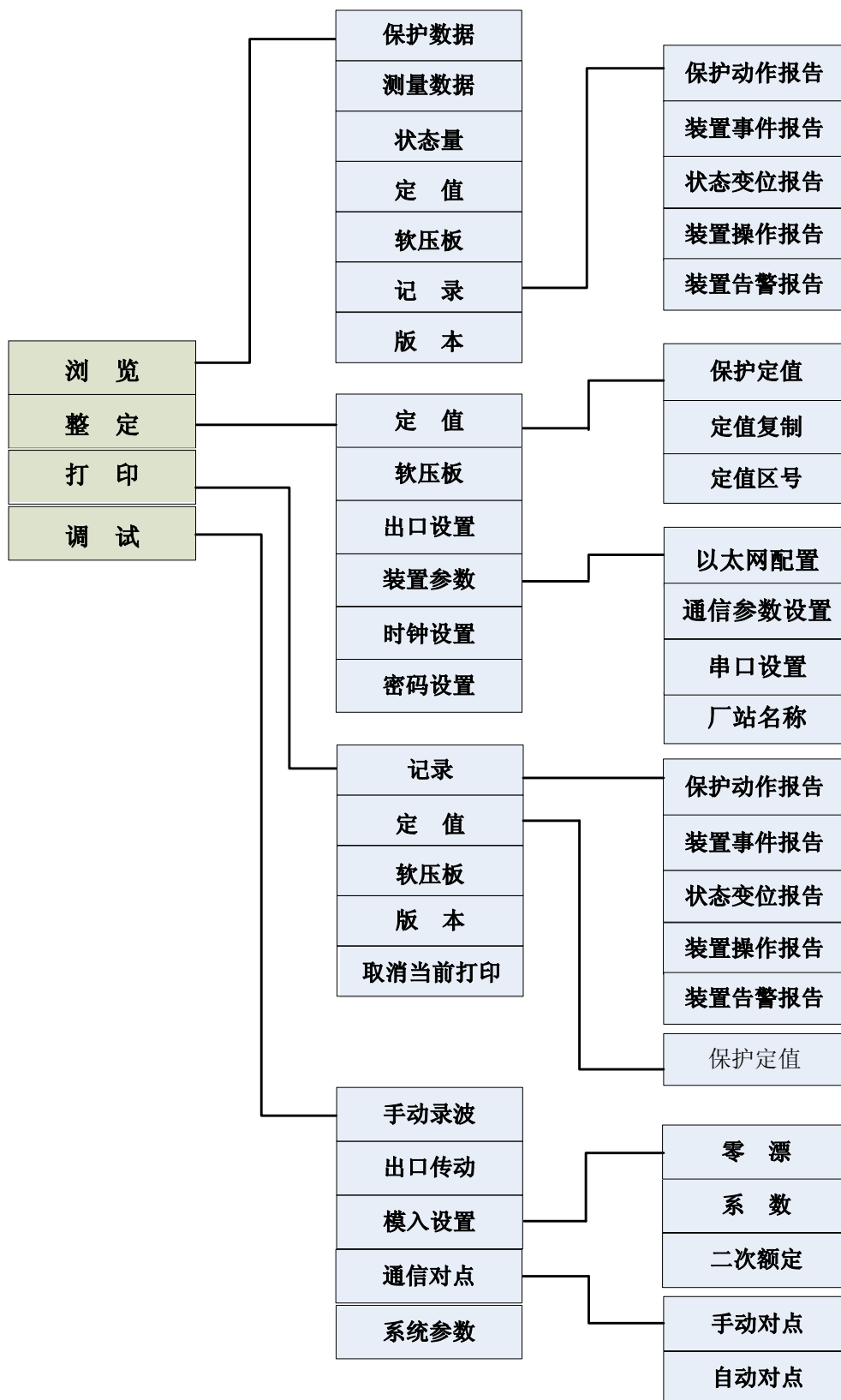
图 6-3-1 菜单结构图
