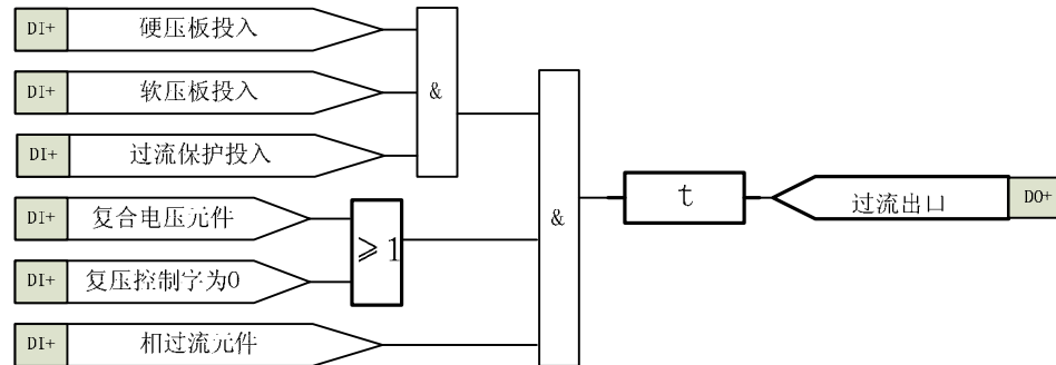
图 4-4 （复压）过流保护逻辑框图
