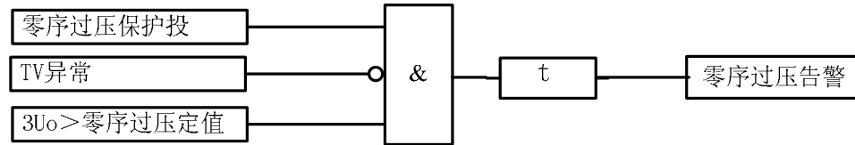
图 4-10 零序过压保护逻辑
