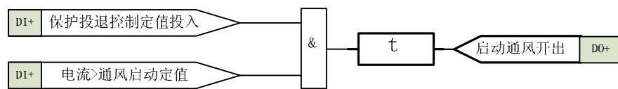
图 4-7 通风启动保护逻辑框图
