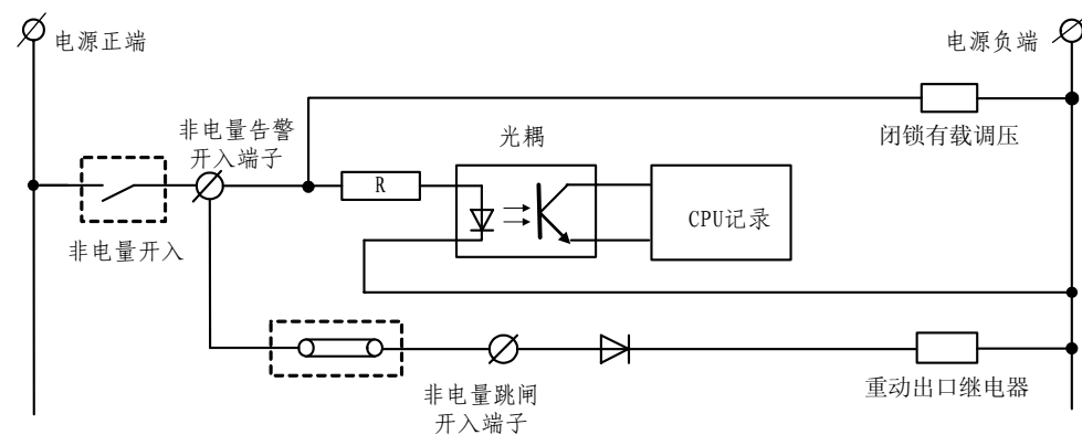
图 4-9 非电量保护逻辑框图
