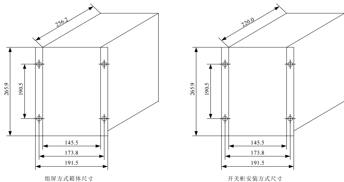
图 3-1 外形尺寸
