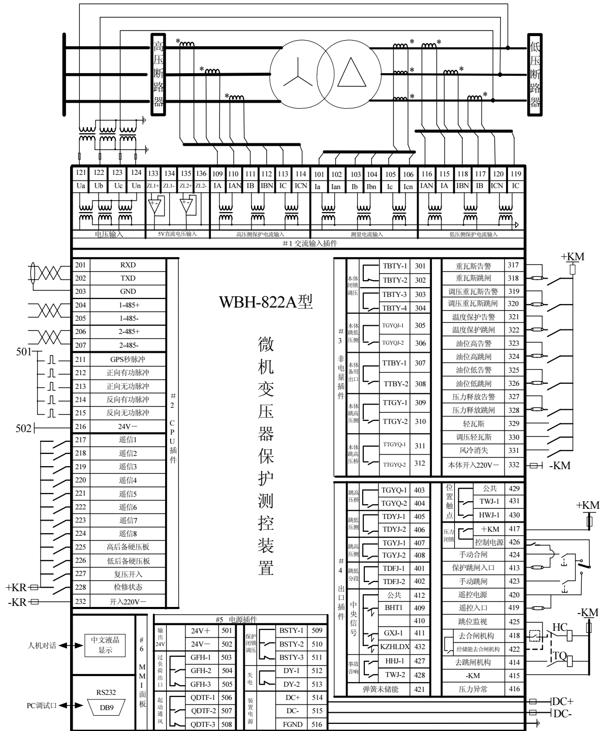
图 12-1 WBH-822A 装置接线示例图
