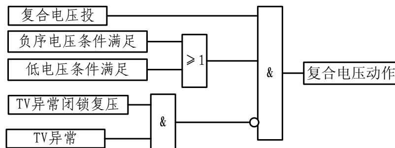
图 4-2 复合电压逻辑图
