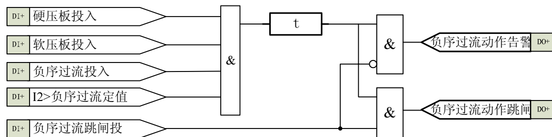
图 4-5 负序电流保护逻辑框图
