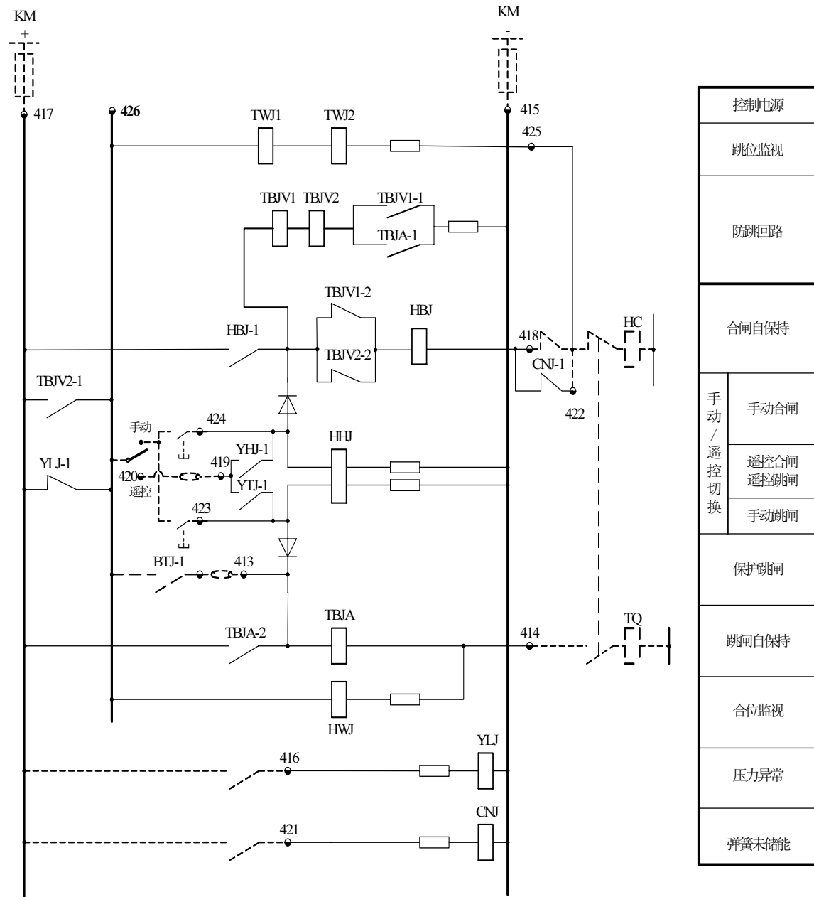
图 12-2 装置操作回路原理图
