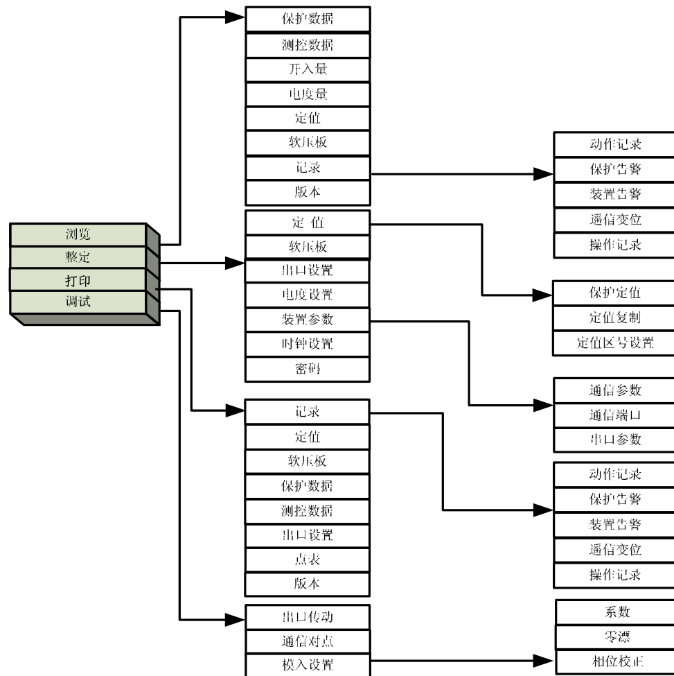
图 5-4 菜单树形结构
