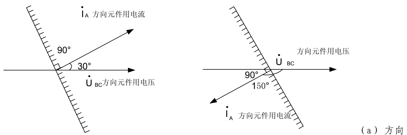
指向变压器时的动作区(阴影侧) (b) 方向指向母线时的动作区(阴影侧)
