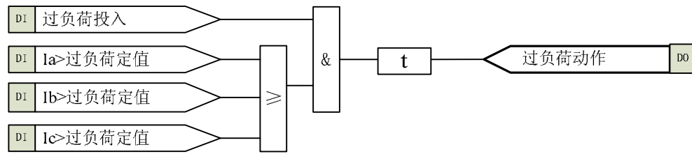
图 4-6 过负荷保护逻辑框图
