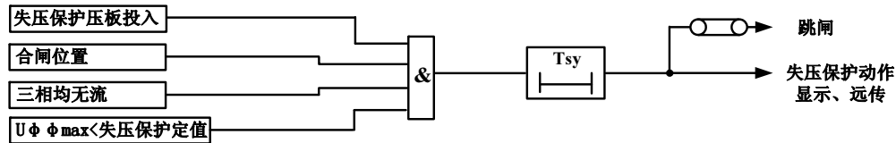
图 3-14 失压保护原理框图
