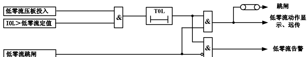
图 3-10 低压侧零序过流保护原理框图
