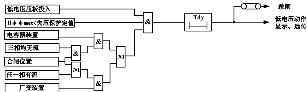
图 3-15 低电压保护原理框图
