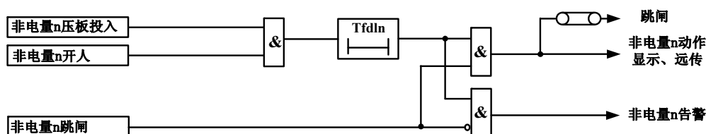
图 3-20 非电量保护原理框图
