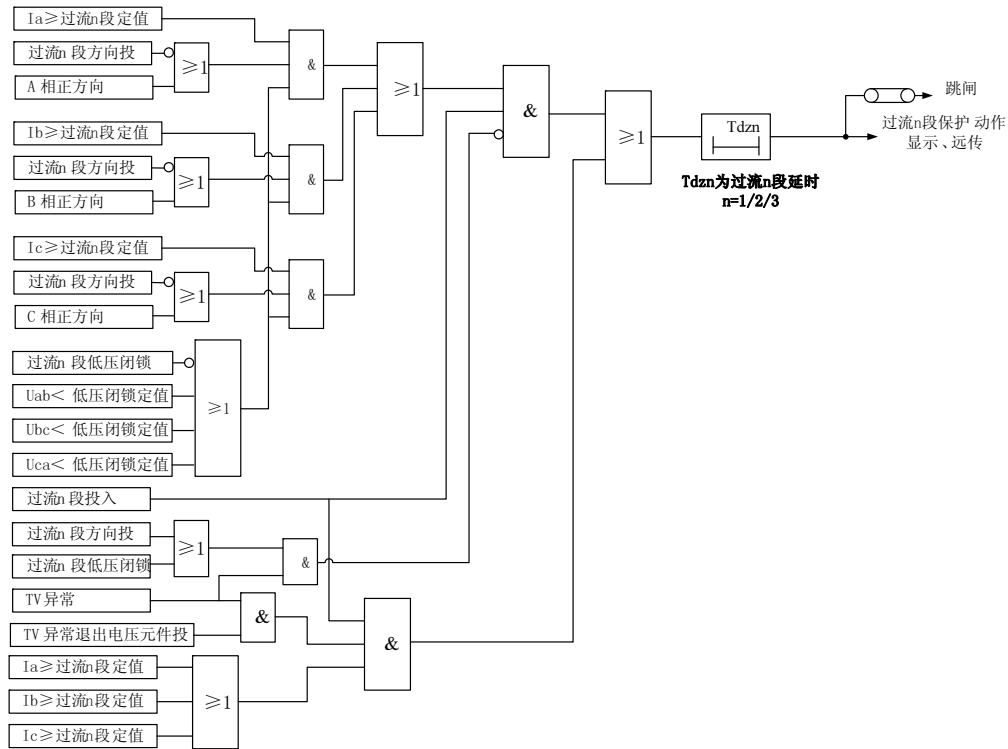
图 3-2 方向（低压）闭锁过流保护原理框图
