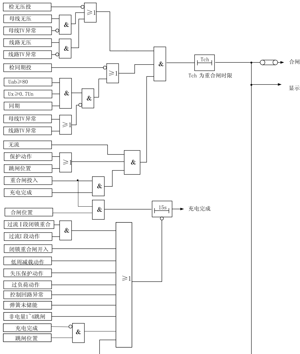
图 3-7 三相一次重合闸原理框图
