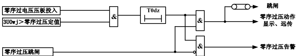
图 3-18 零序过压保护原理框图
