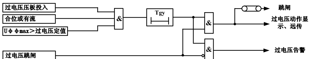
图 3-12 电容器装置过电压保护原理框图
