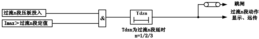
图 3-4 过流保护原理框图
