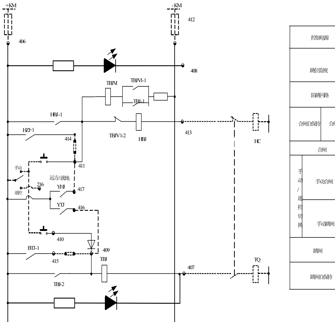
装置操作回路原理图
