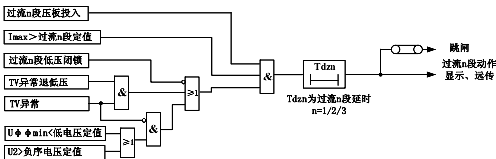
图 3-3 复压闭锁过流保护原理框图
