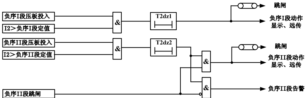
图 3-8 负序过流保护原理框图
