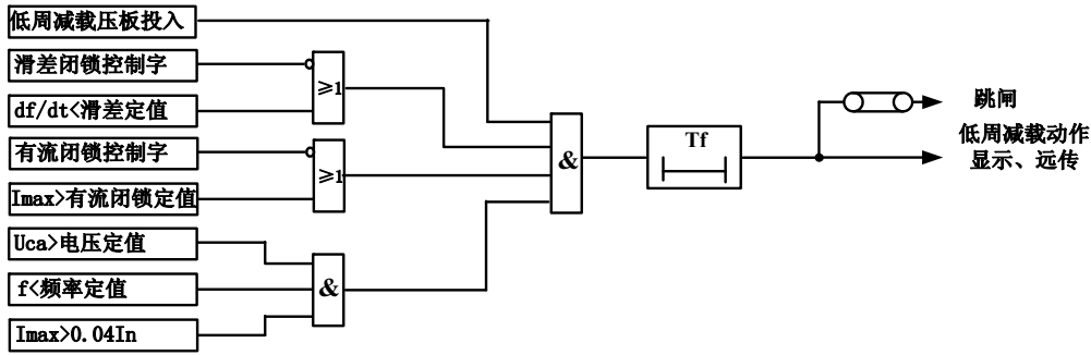
图 3-13 低周减载原理框图
