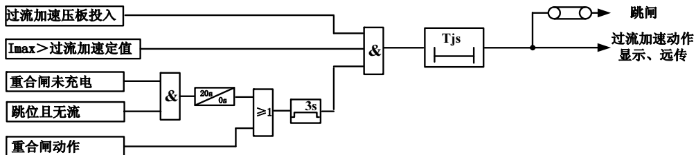
图 3-6 加速保护原理框图
