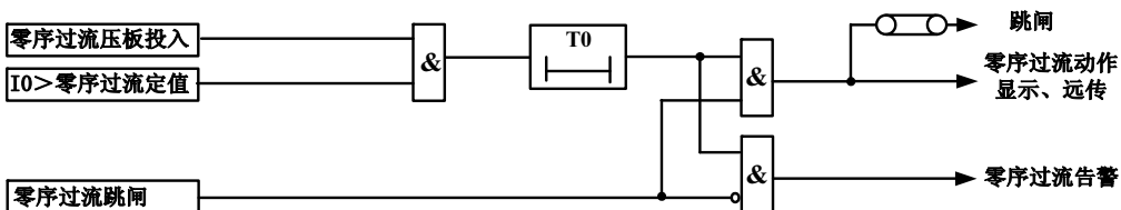
图 3-9 零序过流保护原理框图
