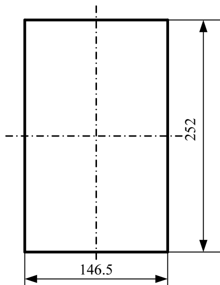
图 7-2 安装开孔尺寸
