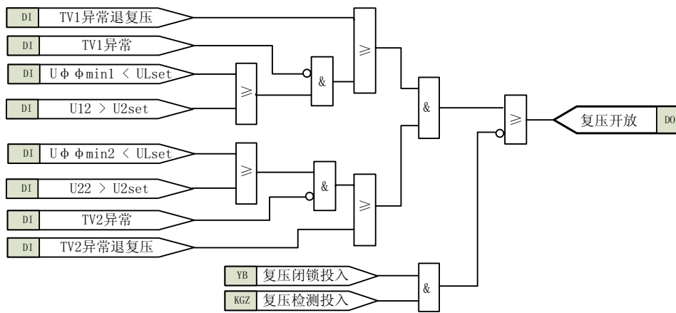
图 3-9 复压闭锁原理框图
