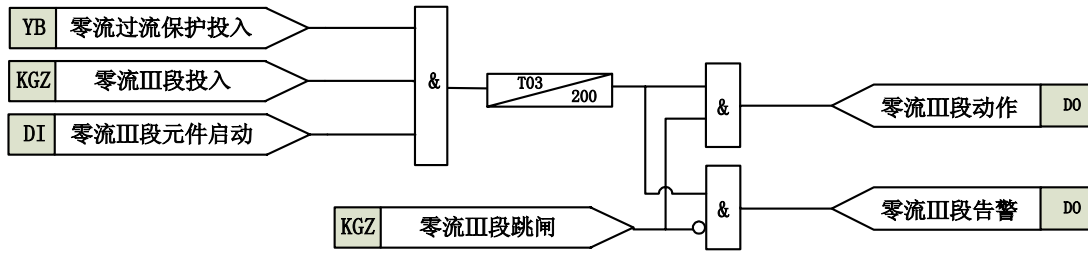
图 3-5 零序过流保护原理框图 2
