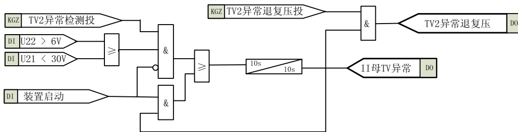
图 3-7 II 母 TV 异常检测原理框图
