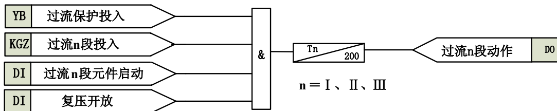
图 3-3 过流保护原理框图
