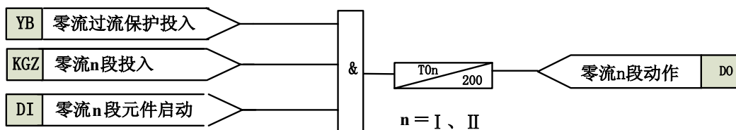
图 3-4 零序过流保护原理框图 1
