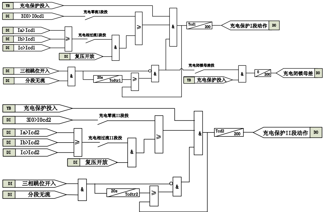
图 3-2 充电保护原理框图
