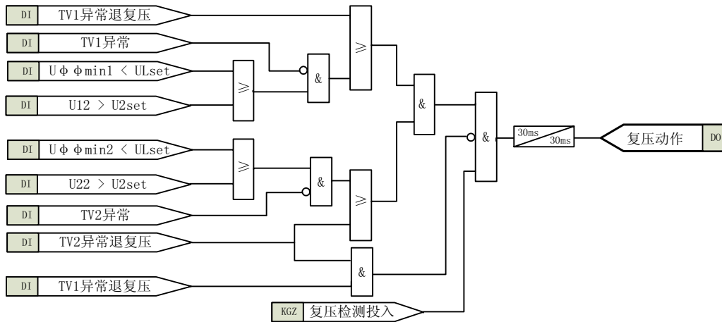
图 3-8 复压动作原理框图
