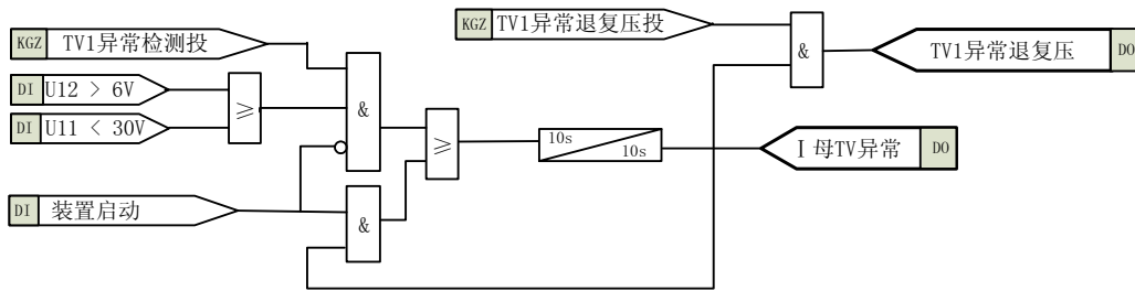
图 3-6 I 母 TV 异常检测原理框图
