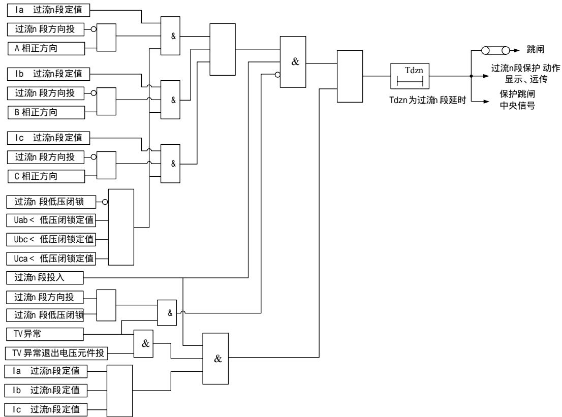
图 3-2：过流保护原理框图
