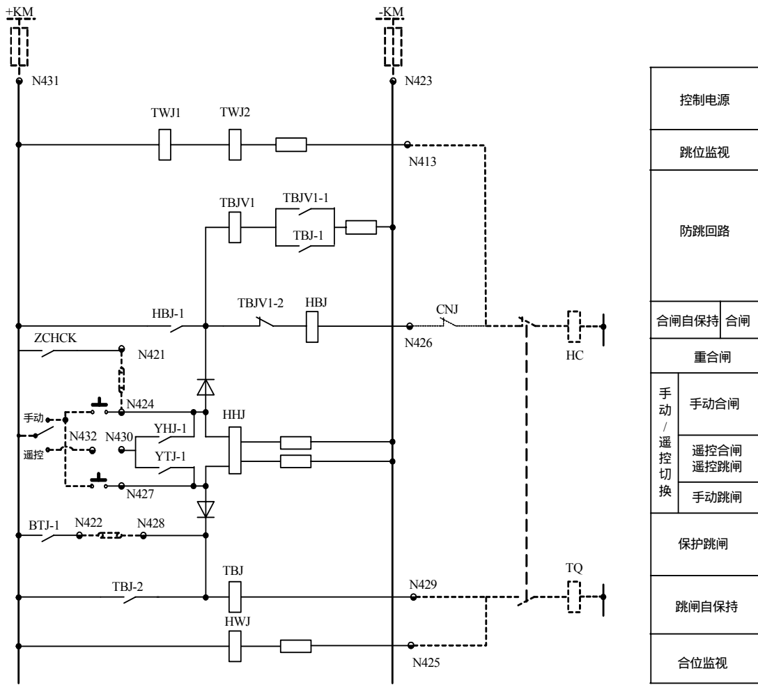
图 12-4：装置操作回路原理图
