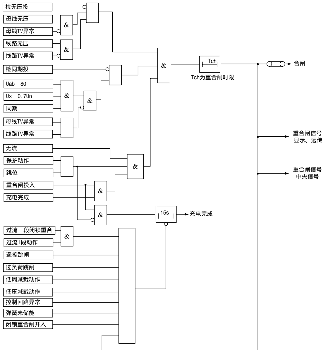
图 3-9 三相一次重合闸原理框图
