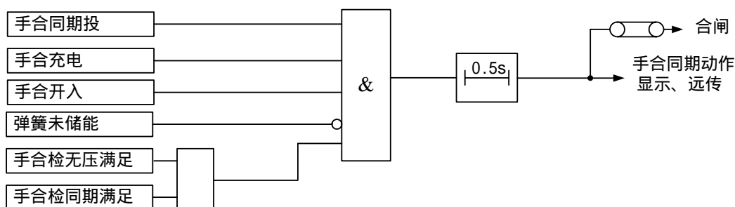
图 3-10 手合同期原理框图
