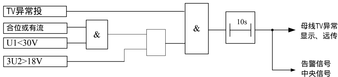
图 3-11 TV 异常检测原理框图
