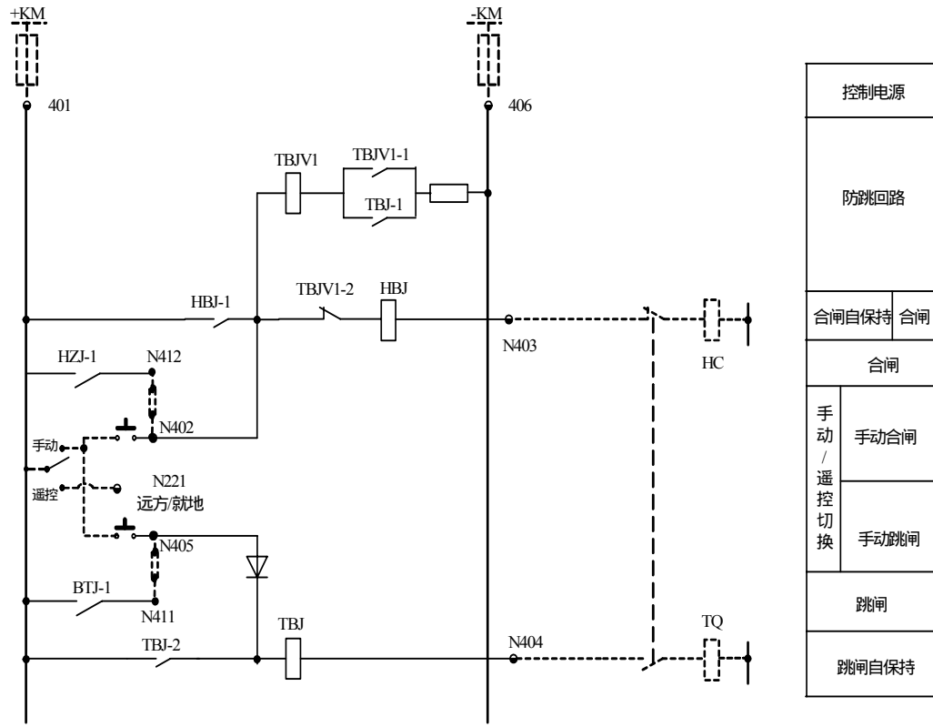
图 12-2：装置操作回路原理图
