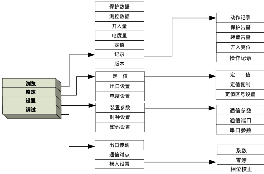
图 4-4 菜单树形结构
