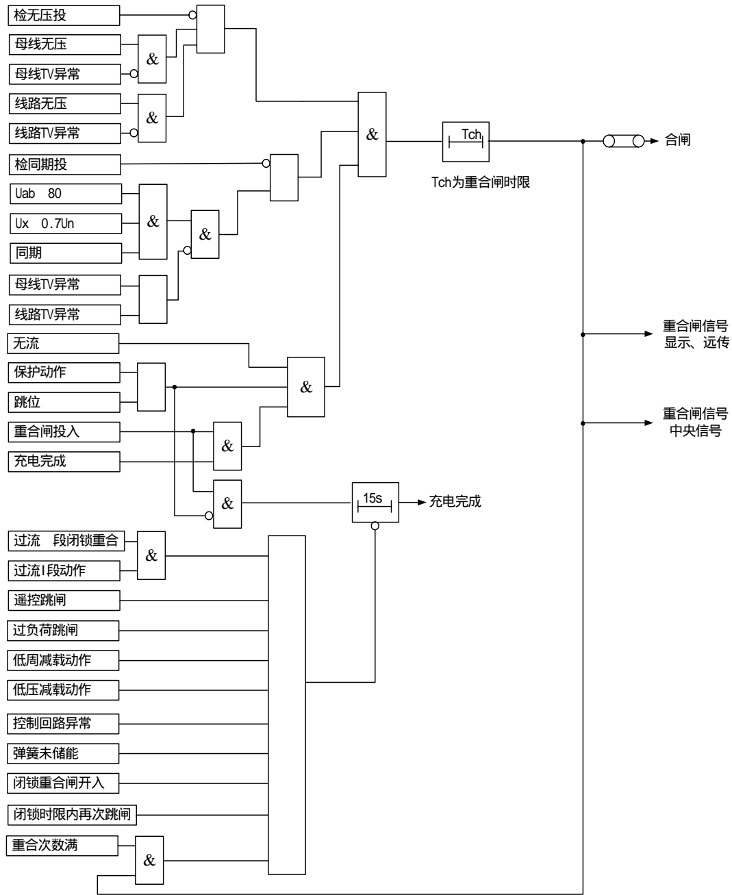
图 3-8 三相多次重合闸原理框图
