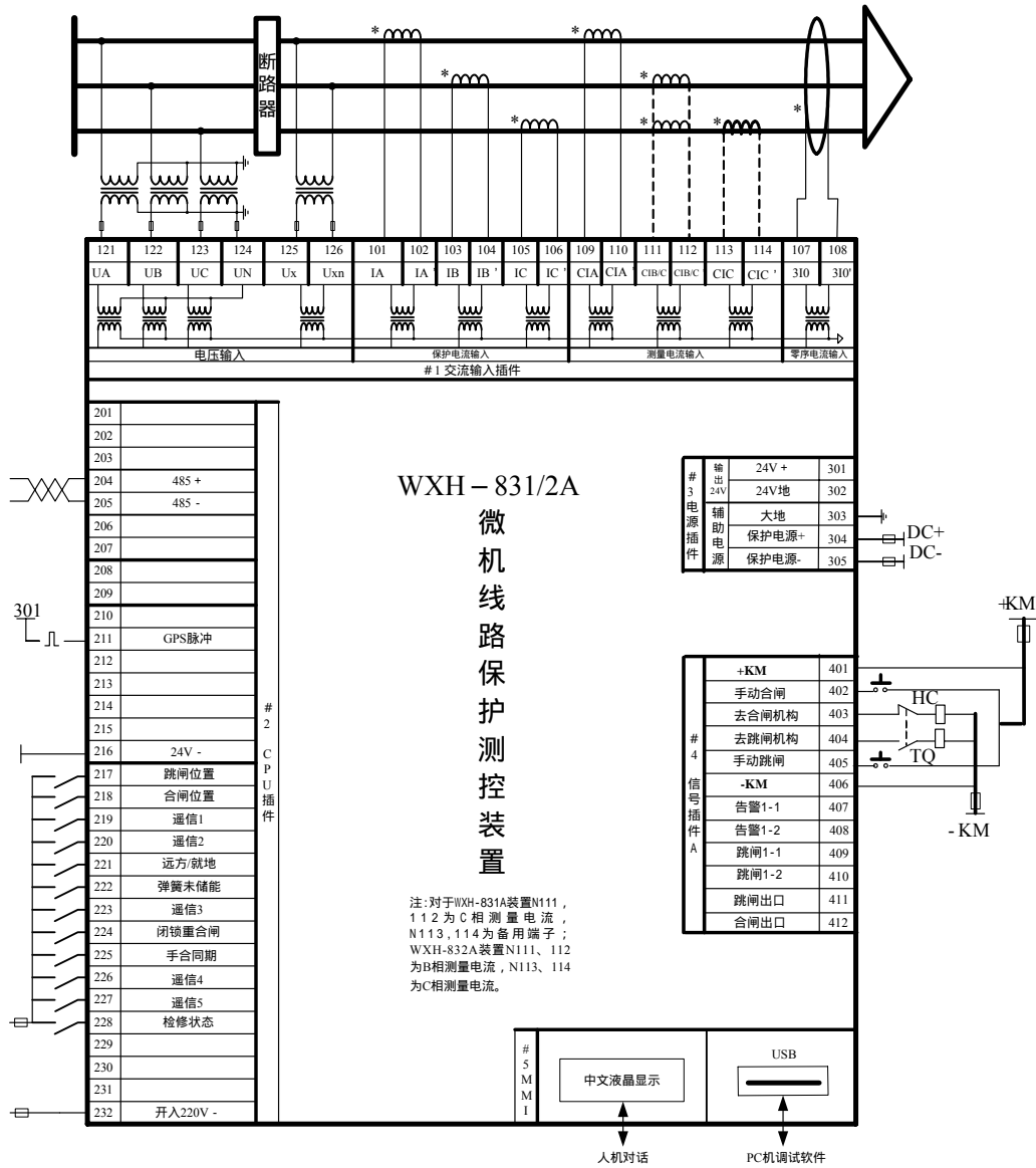
图 12-1：装置接线示意图
