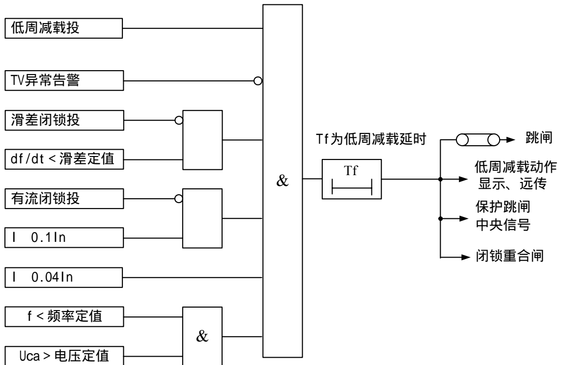
图 3-6 低周减载原理框图
