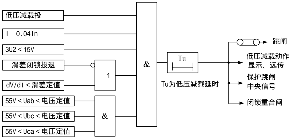
图 3-7 低压减载原理框图
