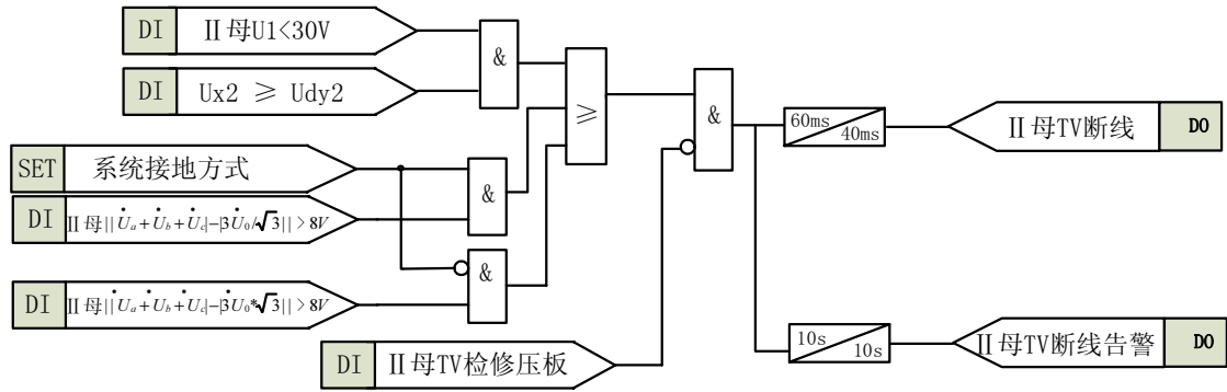
图 3-5 TV 断线检测原理框图
