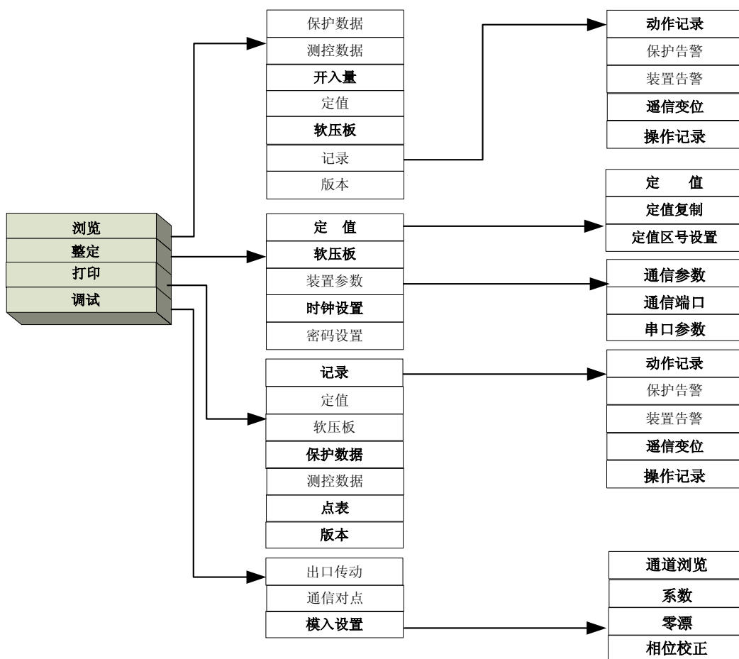
图 4-4 菜单树形结构
