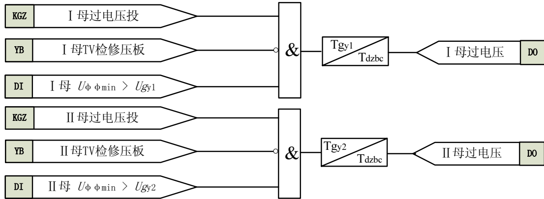
图 3-3 过电压告警原理框图
