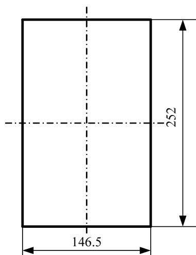
图 2-2 安装开孔尺寸
