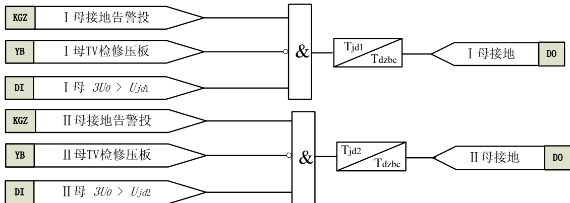
图 3-4 接地告警原理框图
