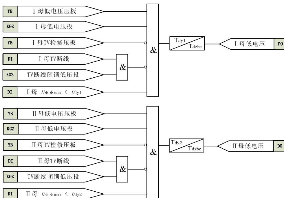
图 3-2 低电压告警原理框图
