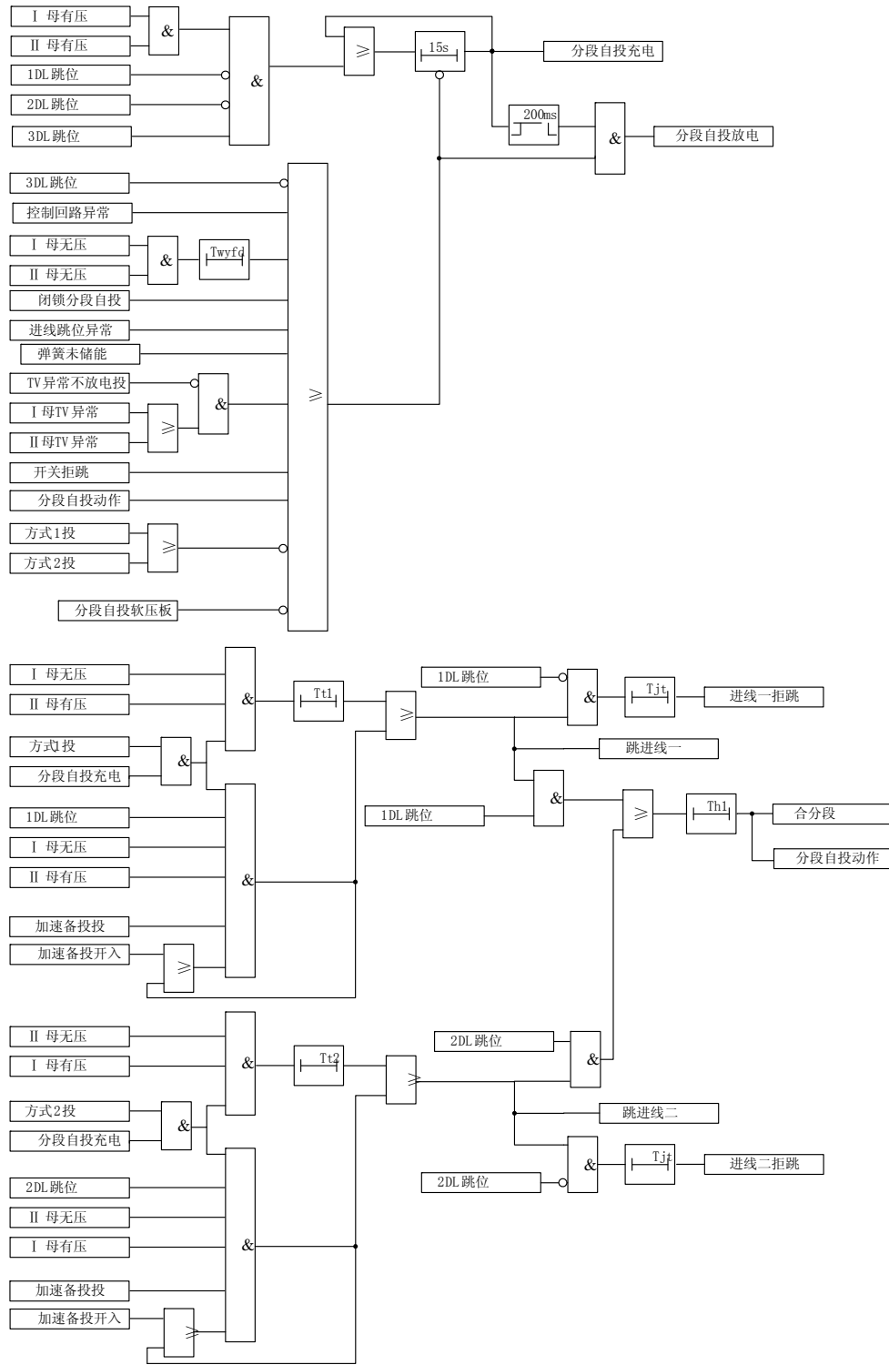
图 3-2 分段备自投逻辑框图
