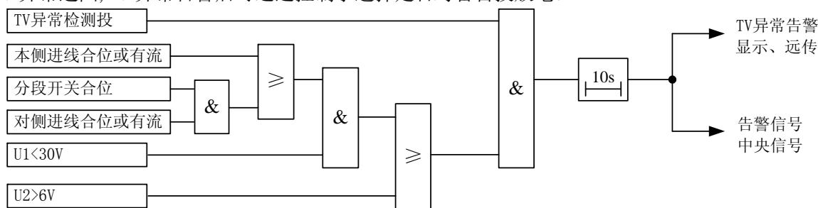
图 3-3 TV 异常检测原理框图
