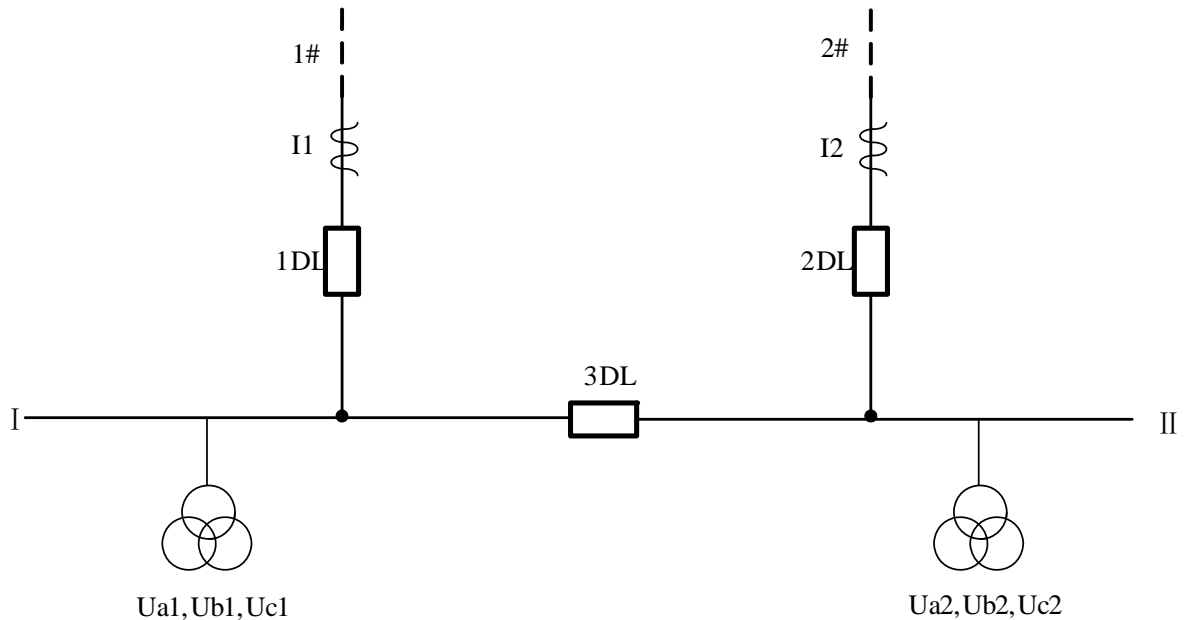
图 3-1 运行方式接线图
